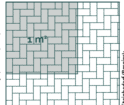
Steinbedarf (Besoins): 20 x 10 cm je (par) m 2 - 50 St. (pièces)
