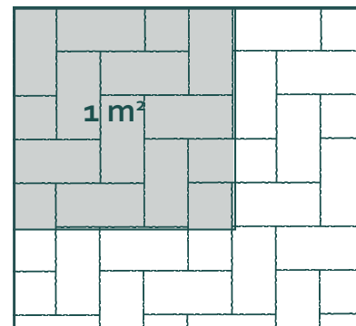
Steinbedarf (Besoins): 20 x 40 cm je (par) m 2 - 12,5 St. (pièces)
